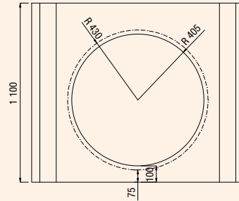
Regard EP | 300 x | 300
